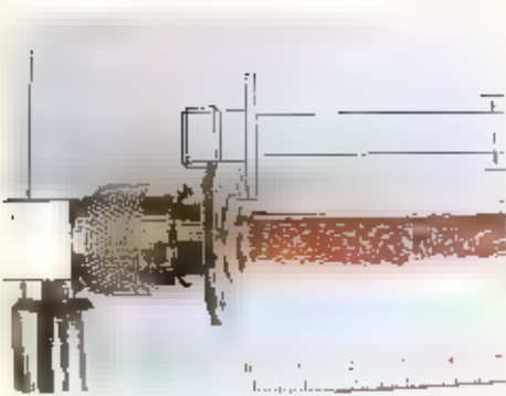
Koperfolie om de teflontape heen gevouwen. Soldeer de folie aan de folie van de mantel en de massa van de N connector vast.
